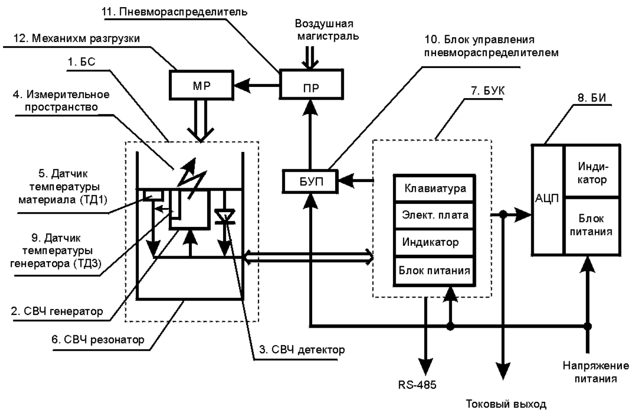
Рис. 6.3. Функциональная схема влагомера «Микрорадар-114А(D)13Р»
