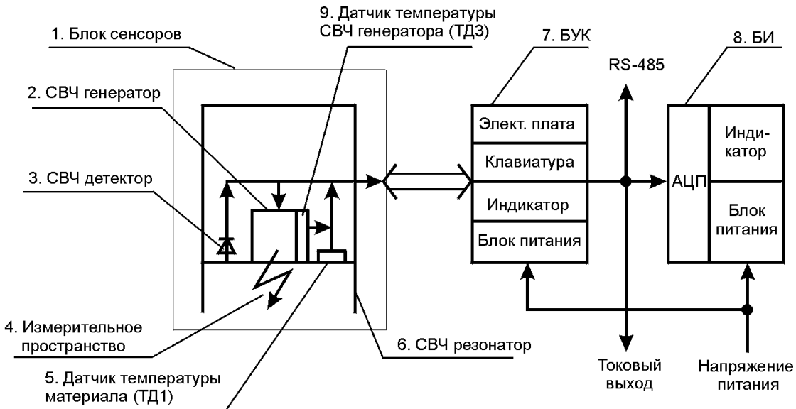
Рис. 6.1. Функциональная схема влагомеров «Микрорадар-114А(D)13К» и «Микрорадар-114А(D)13В»
